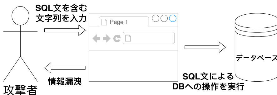
図 3.2: SQL インジェクション攻撃の例
