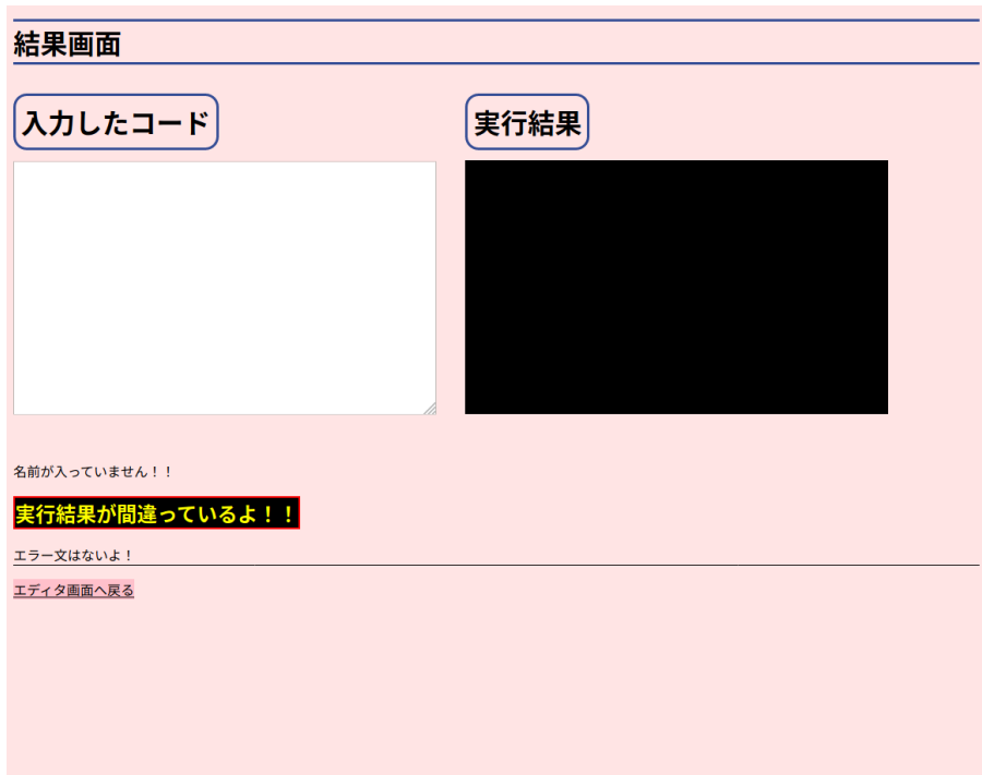
図 6.2: 実行ページ
